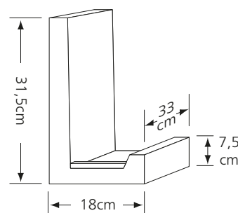
KSZTAŁTKA WIEŃCOWA KLBL 24
