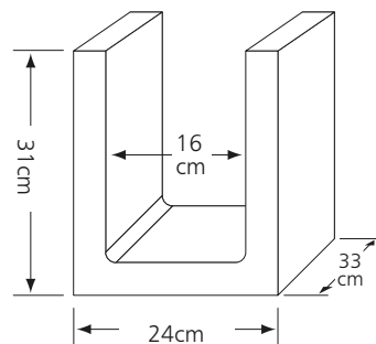
KSZTAŁTKA ŻEBRA ROZDZIELCZEGO UZUPEŁNIAJĄCA 30
