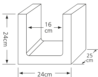
KSZTAŁTKA ŻEBRA ROZDZIELCZEGO 70EU
