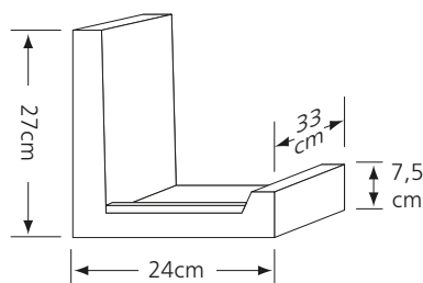
KSZTAŁTKA WIEŃCOWA KLBL 36,5
