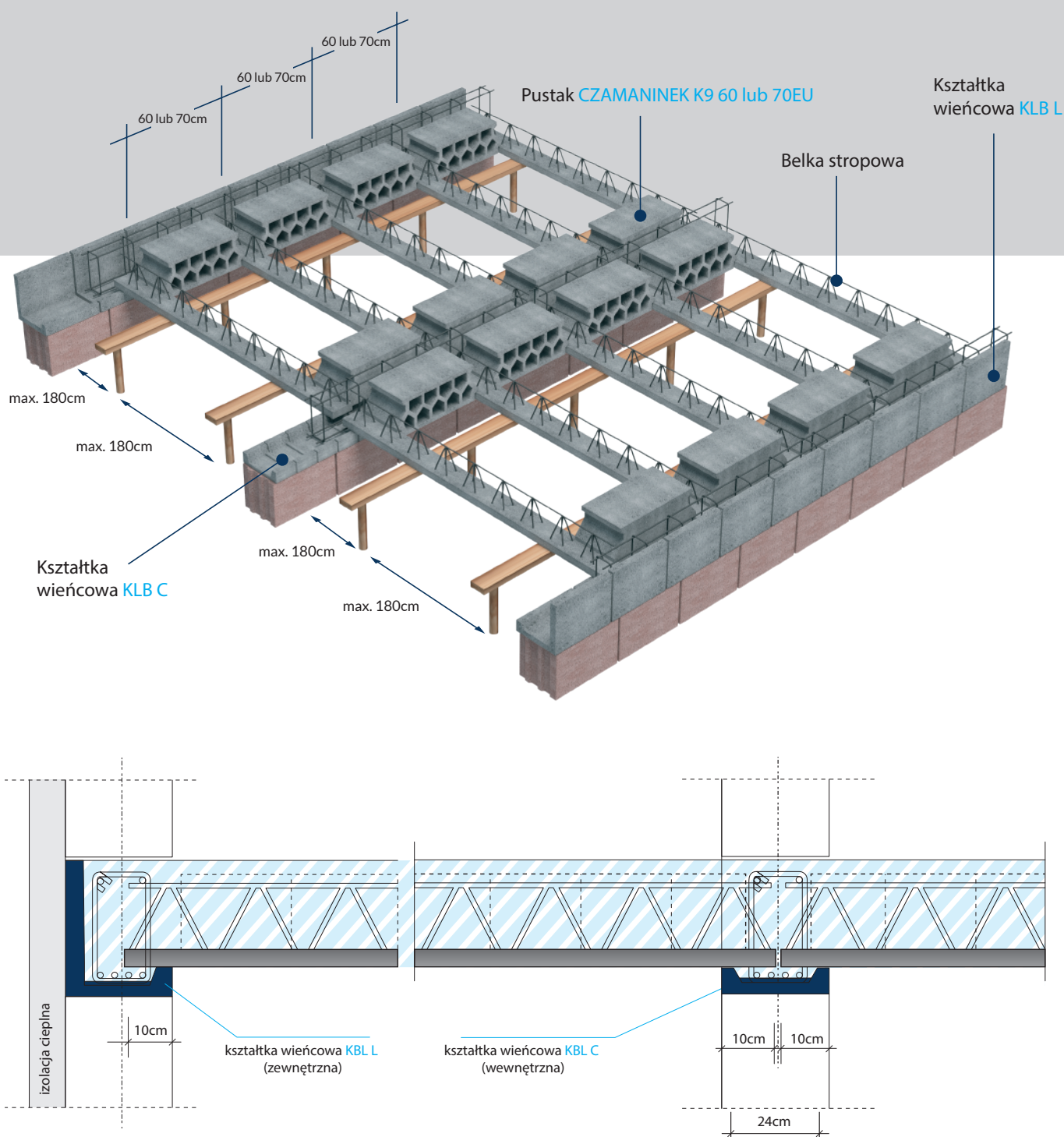
Rys.1 . Strop oparty na ścianie dwuwarstwowej i wewnętrznej z wykorzystaniem kształtek KLB L i KLB C.
