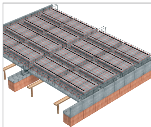
Łączenie siatek 15x15 lub 20x20 na zakładkę (jedno oczko)
