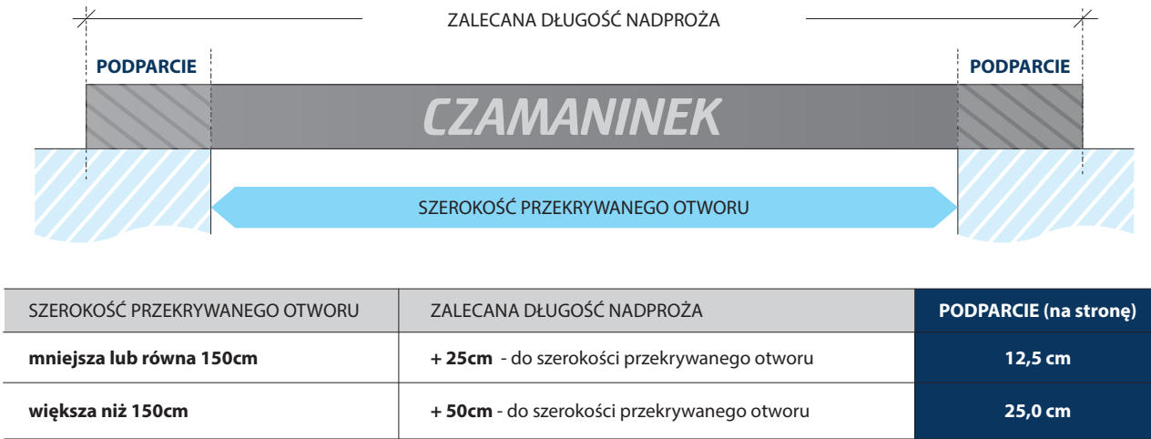
Rys. 10 - PODPIERANIE NADPROŻY BEZPOŚREDNIO NA MURZE - prawidłowy dobór długości nadproża
