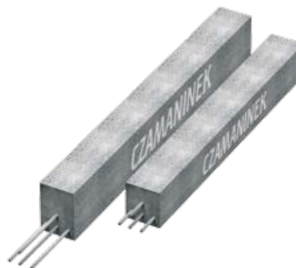
NADPROŻA SPRĘŻONE 14,0 x 11,0 i 11,0 x 11,0
